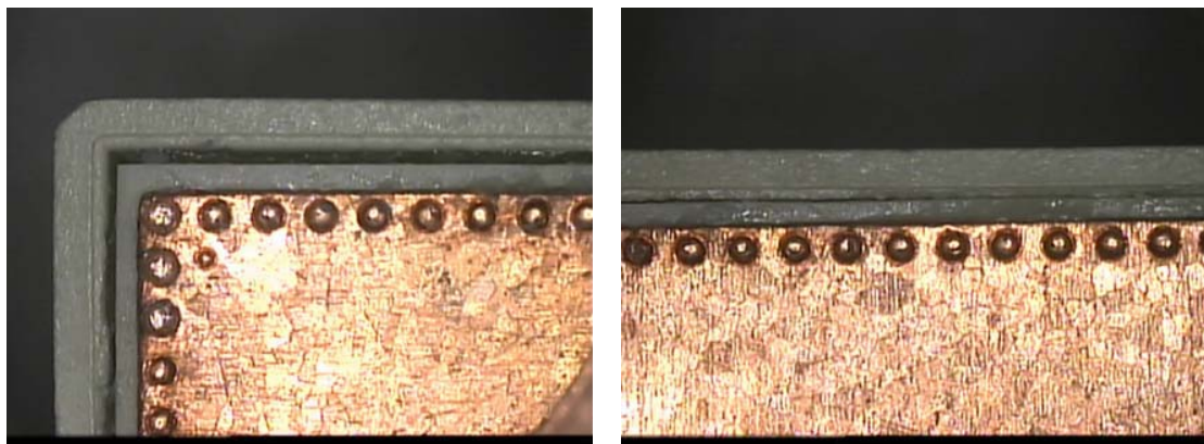
Fig. 6: Dimples in MiniSKiiP bottom surface Abb. 6: Geätzte Vertiefungen auf der MiniSKiiP Unterseite
